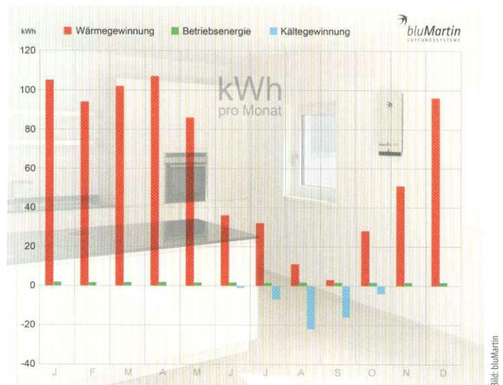
bluMartin: „Kältegewinnung“ mit freeAir 100.
