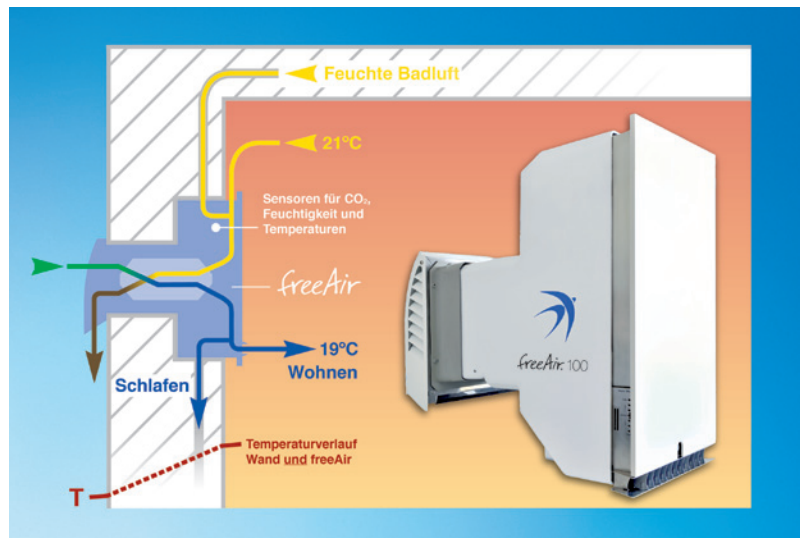
Das Funktionsprinzip eines dezentralen Lüftungsgeräts
