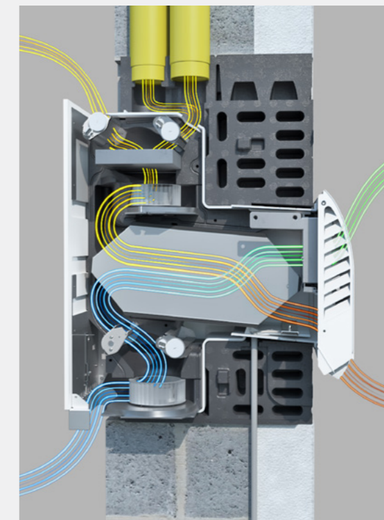
Sezione freeAir 100 e con scambiatore di calore in controcorrente a flusso incrociato
